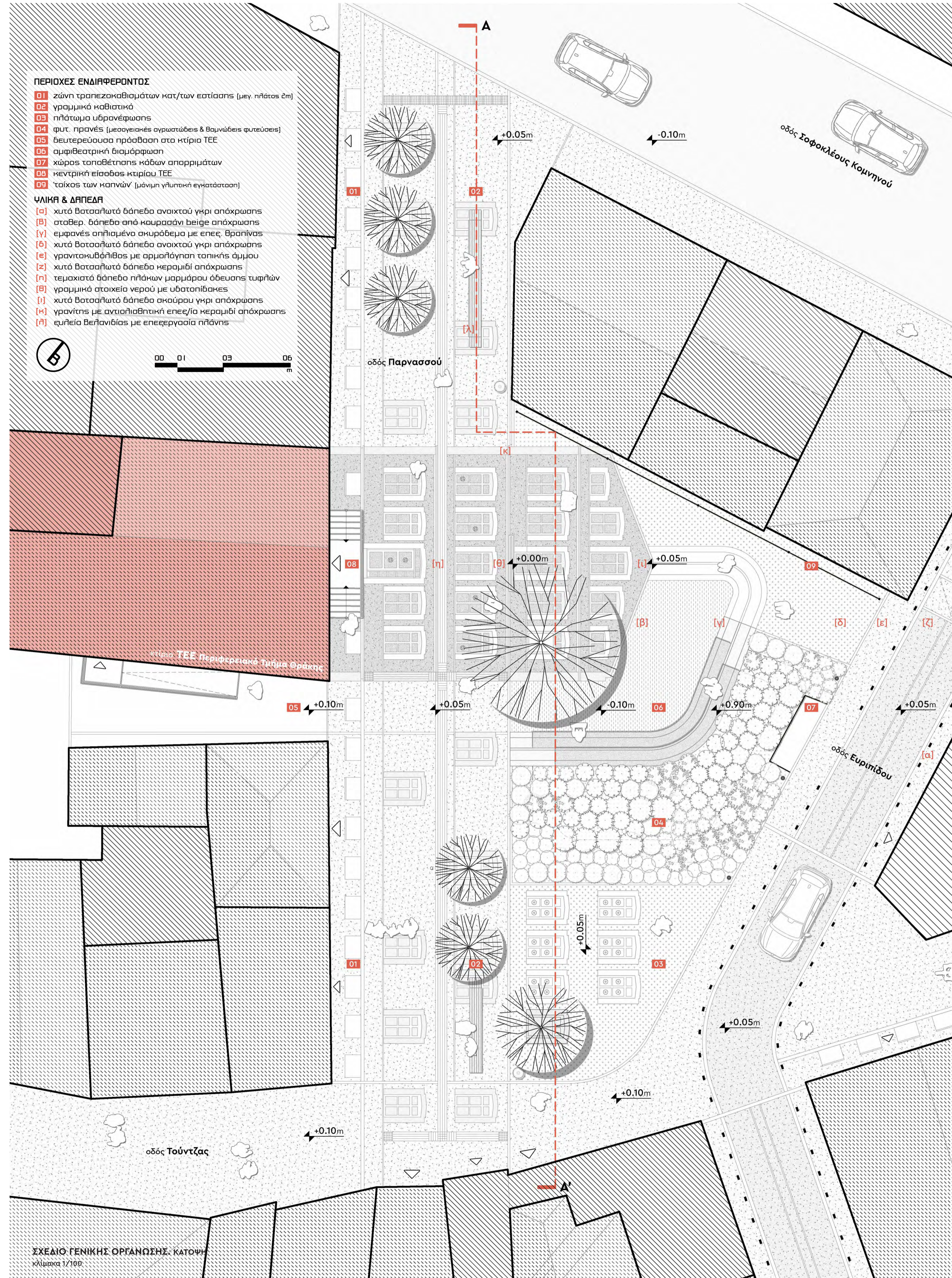
ΑΣΤΙΚΟΙ ΥΠΑΙΘΡΙΟΙ ΧΩΡΟΙ & ΝΕΟΤΕΡΑ ΙΣΤΟΡΙΚΑ ΒΙΟΜΗΧΑΝΙΚΑ ΚΤΙΡΙΑ. ΔΙΑΓΡΑΜΜΑ κλίμακα 1/10000
